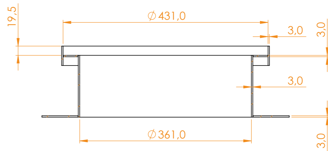
SECTION D-D
